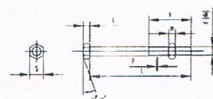
Bolt and Nut สลักเกลียวและแป้นเกลียว
