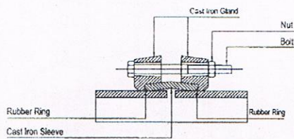
Gibault ข้อต่อยึบดัต
